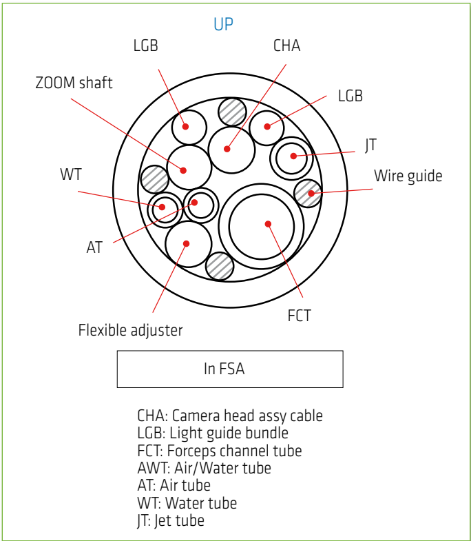
FIGURA 7. Componentes del extremo distal del endoscopio.
